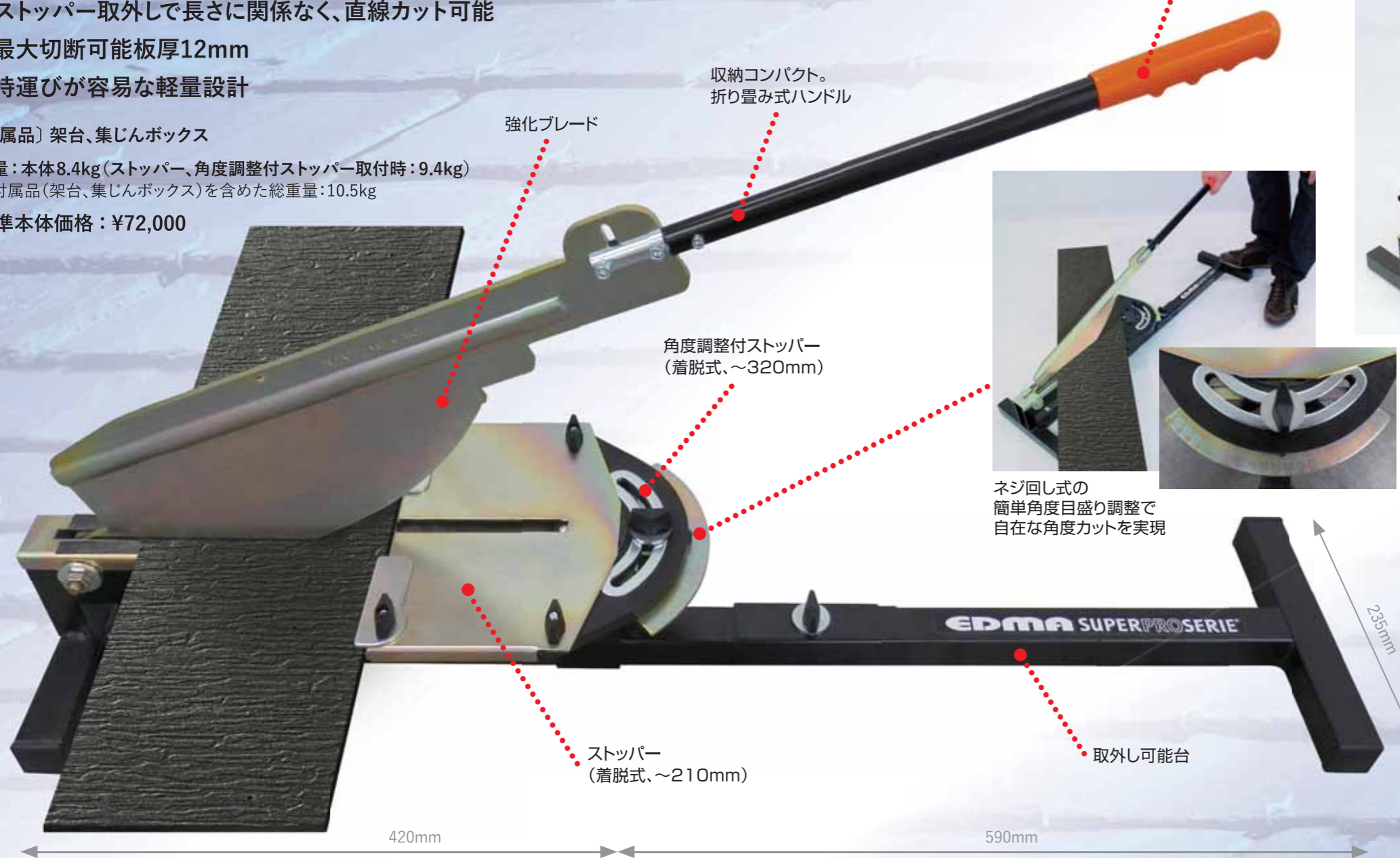
全ストッパー取外しでスレート長に関係なく直線カットが可能
