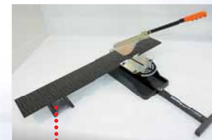
付属の架台で 安定カット
